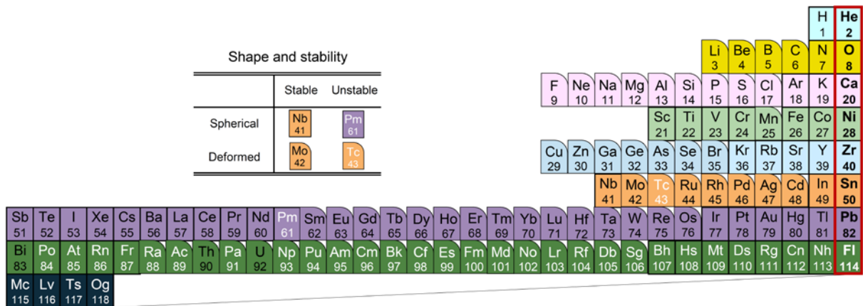
図 1：新しい原子核の周期表
