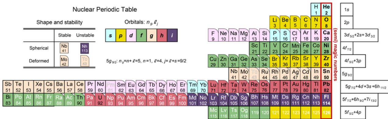
図 4. 陽子の軌道ごとに色分けした原子核の周期表
